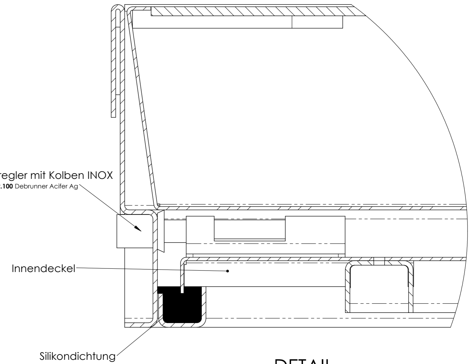
DETAIL C MABSTAB 1 : 1
